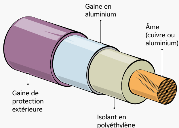
Constitution d'un câble
